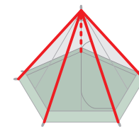
赤で示した各辺をダイニーマ®テープで補強
