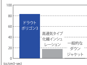
【通気度試験】(当社試験データ)
