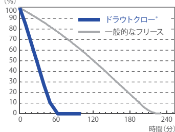
【拡散性残留水分率】(当社試験データ)
