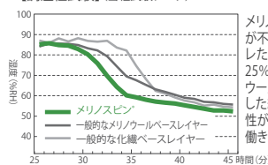
【調湿性試験】(当社試験データ)
