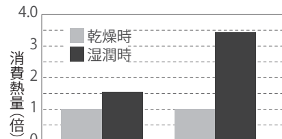
【消費熱量比較テスト】（当社試験データ）
